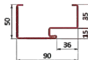
profil ościeznicy do drzwi 55mm FD-21 / B-55
