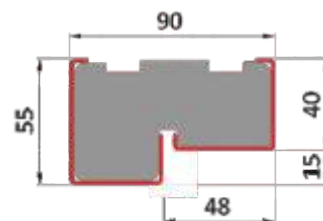
profil ościeznicy do drzwi 72mm stalowo-drewniana - 72
